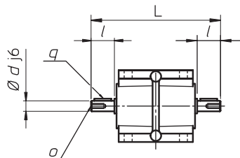
Vers.2 Beidseitige Eintriebswelle
