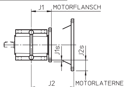
Vers.3 Motorflansch oder Motorlaterne
